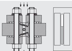
Direction de vision Type de réfraction avec des blindages en mica
