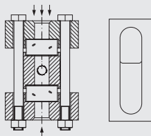
Direction de vision selon DIN 7081
